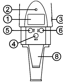
Abbildung 4 Sender
