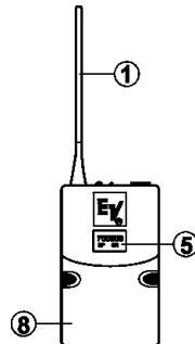
Abbildung 5 Taschensender
